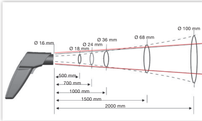
testo 830-T4
