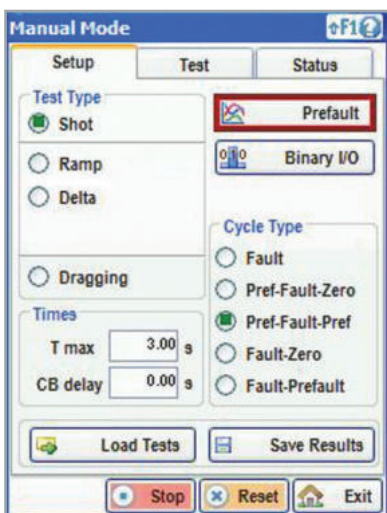
Manueller Prüfaufbau
