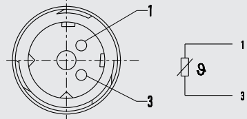
Bajonett-Steckverbinder nach DIN 72585
