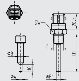
Conector de bayoneta, DIN 72585
