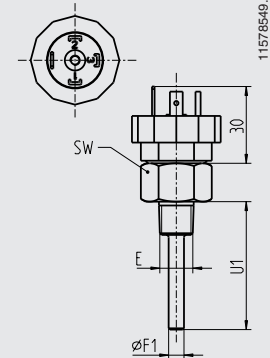
Conector rectangular EN 175301-803, forma A
